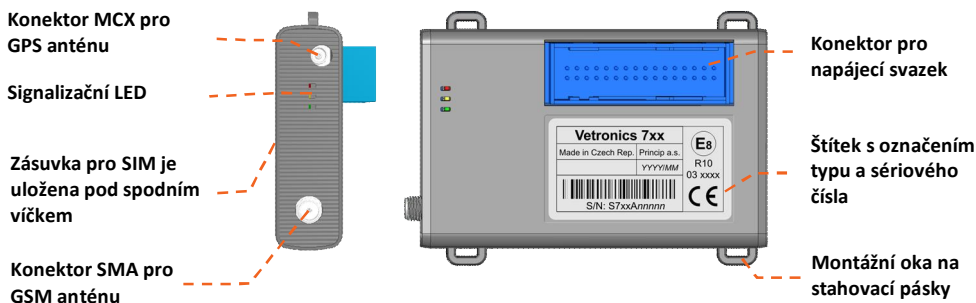
Obrázek 1: rozmístění konektorů na jednotce, pohled z boku a ze shora
